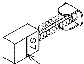
摩耗限界線
